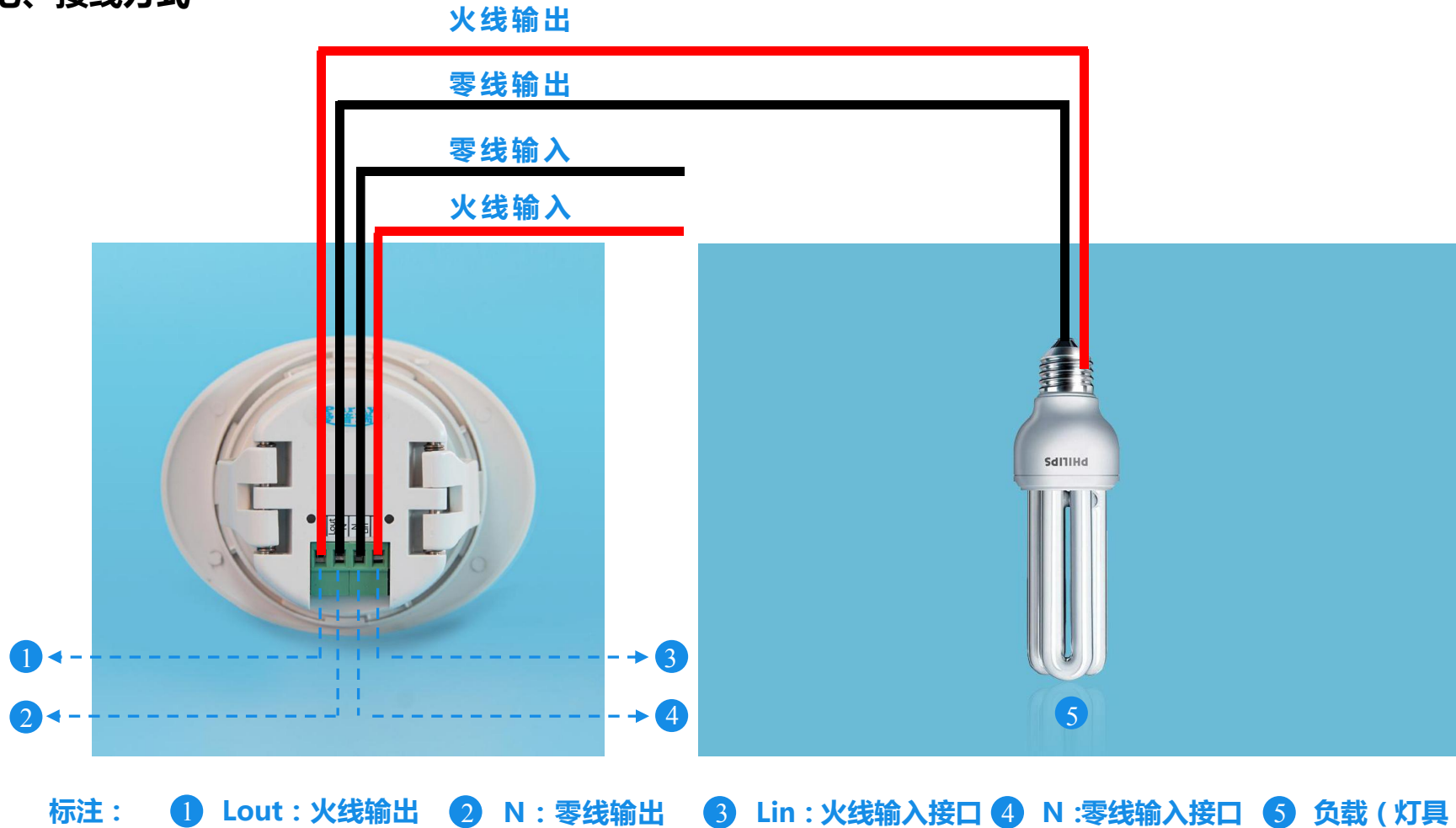
图九 BRT-880 接线方式
