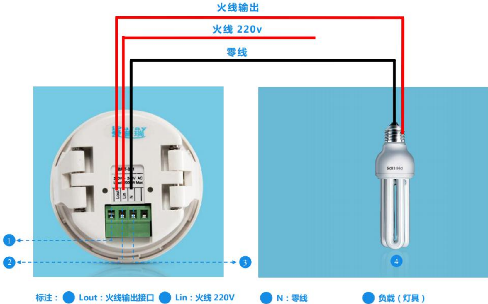
图九 BRT-881 接线方式
